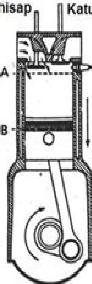
Langkah Hisap
