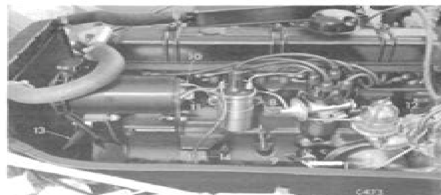
Fig. 2. L.H. side of Vitesse engine
