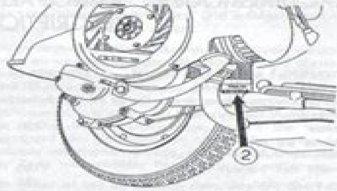
Abb. 2 - Serienbezeichnungen auf Fahrzeugteil (1) und Motor (2).
