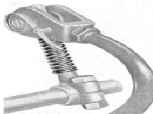
Bild 86. Einbau der Feder Nr. 34395 bei Wagen bis Typ F 7
