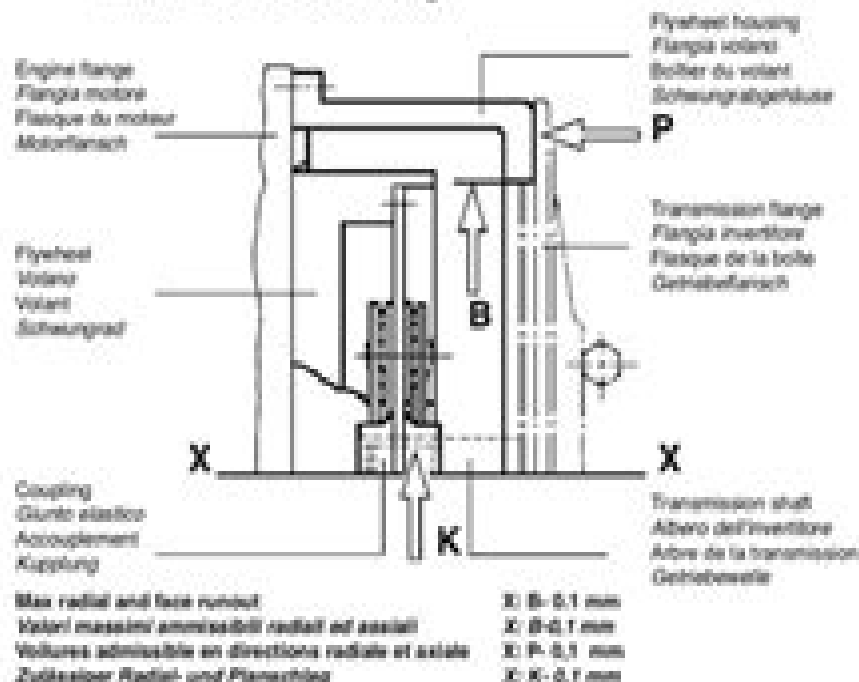
Fig. 4 Engine-transmission connection Accoppiamento trasmissione-asse d'elica Raccordement moteur-boîte Motor-Getriebe-Verbindung
