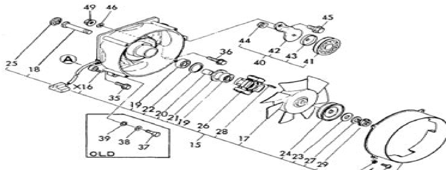
Fig. 10 RADIATOR & FAN
