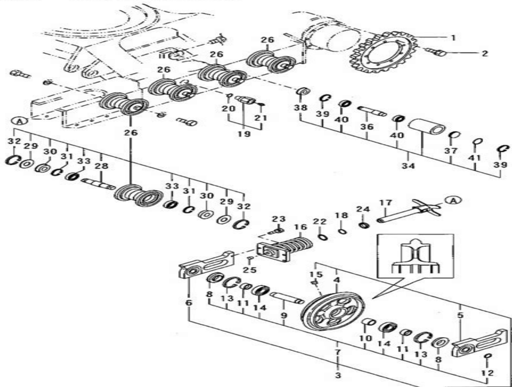
Fig. 1 ROLLER & ADJUST
