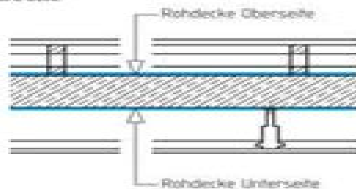
aufgeständerte Fußbodenkonstruktion bzw. abgehängte Decke
