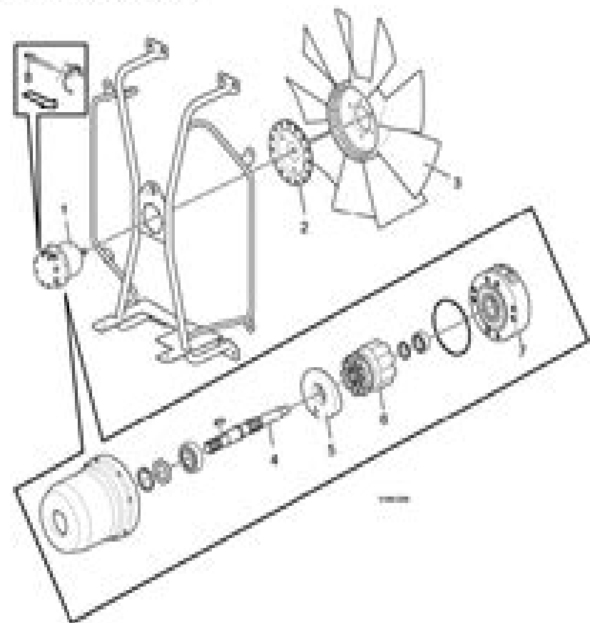
Figure 1 Cooling fan motor and fan
