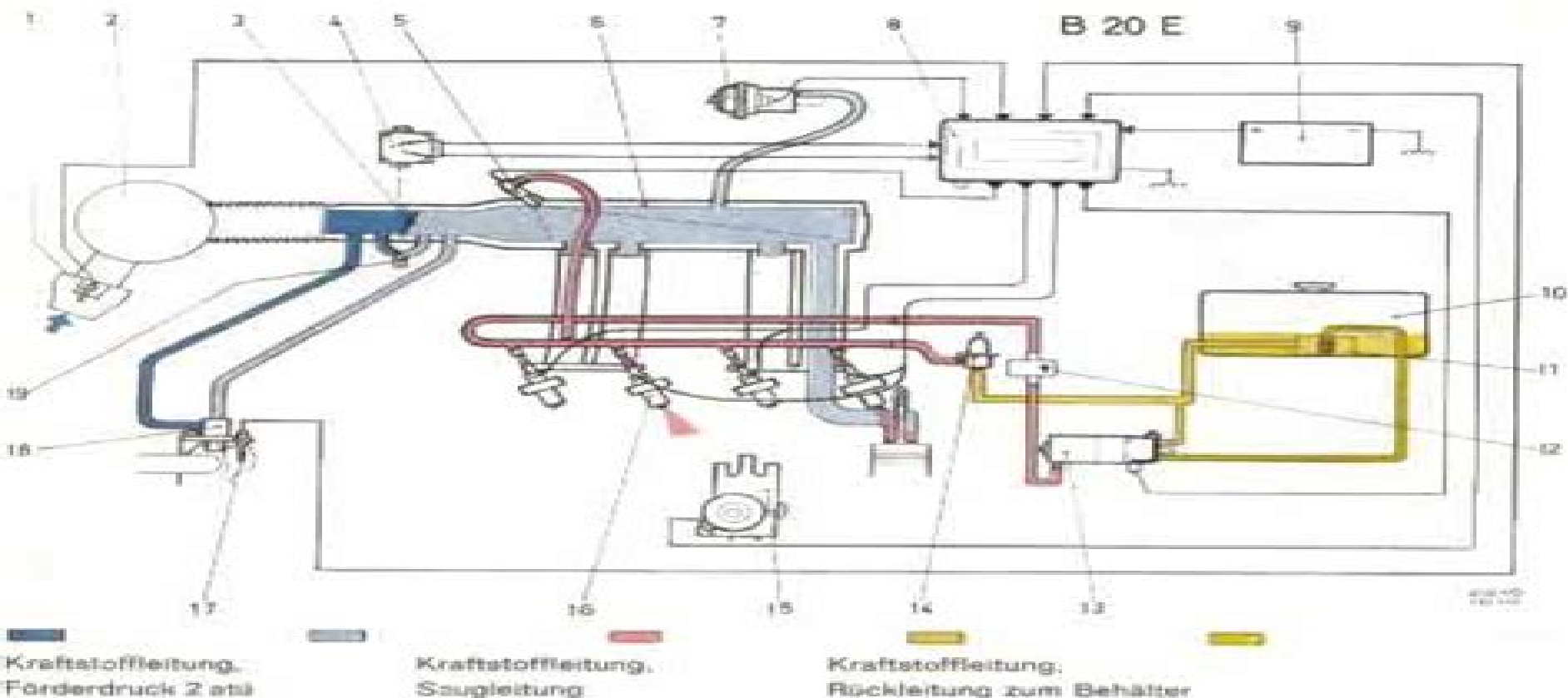
Abb. 2—6 Prinzipskizze über Einspritzanlage, Serie 140
