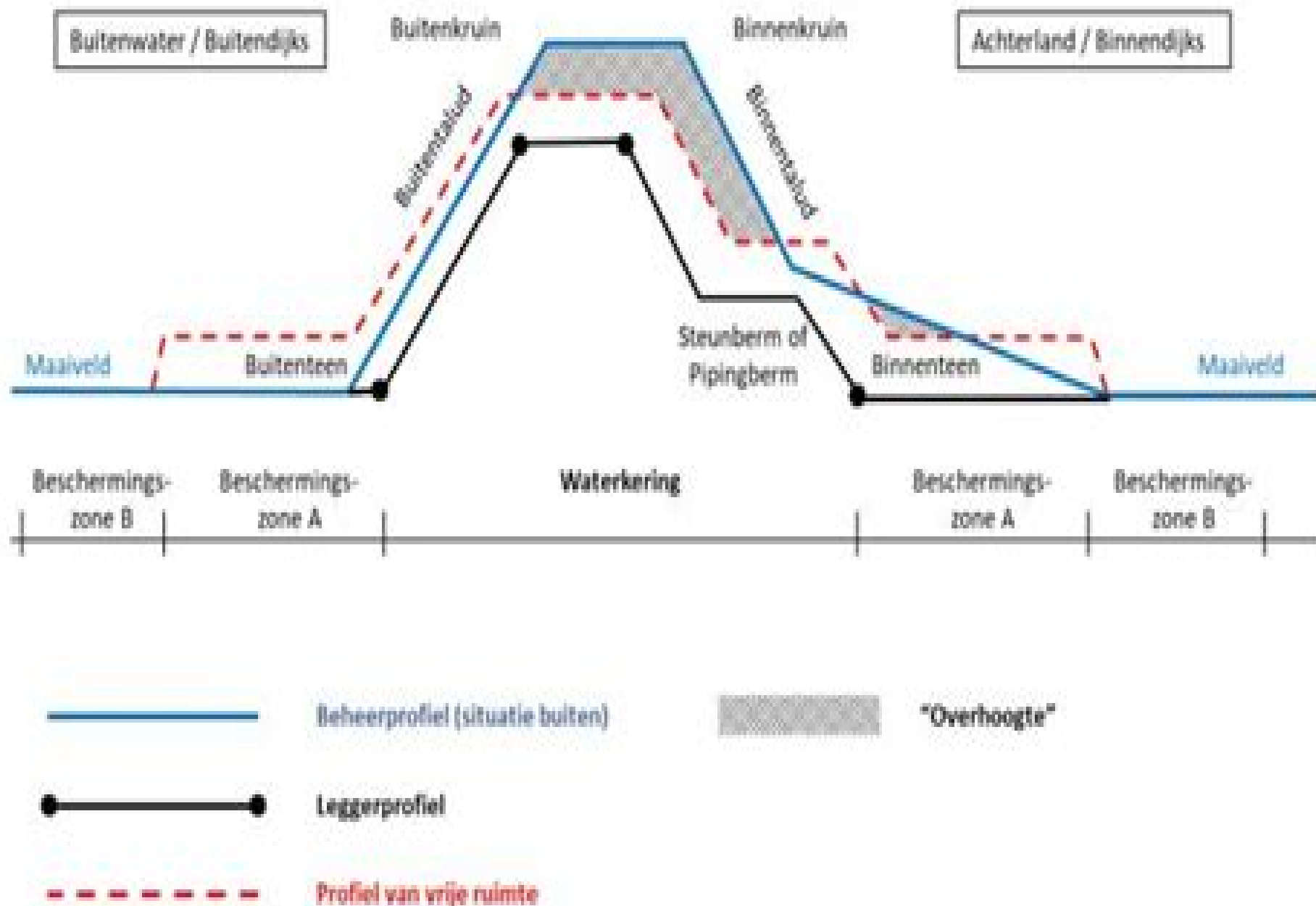
Figuur 17.1: Principeprofiel waterkering met overhoogte
