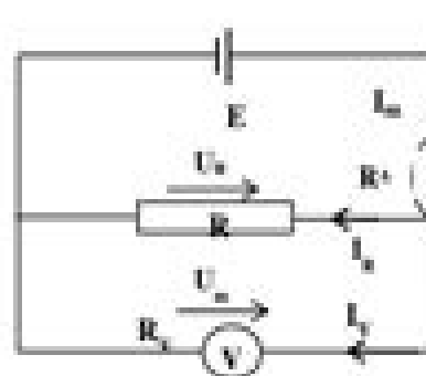
Figure 2 : Montage courte dérivation (ou aval)
