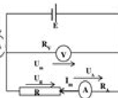
Figure 3 : Montage longue dérivation (ou amont)
