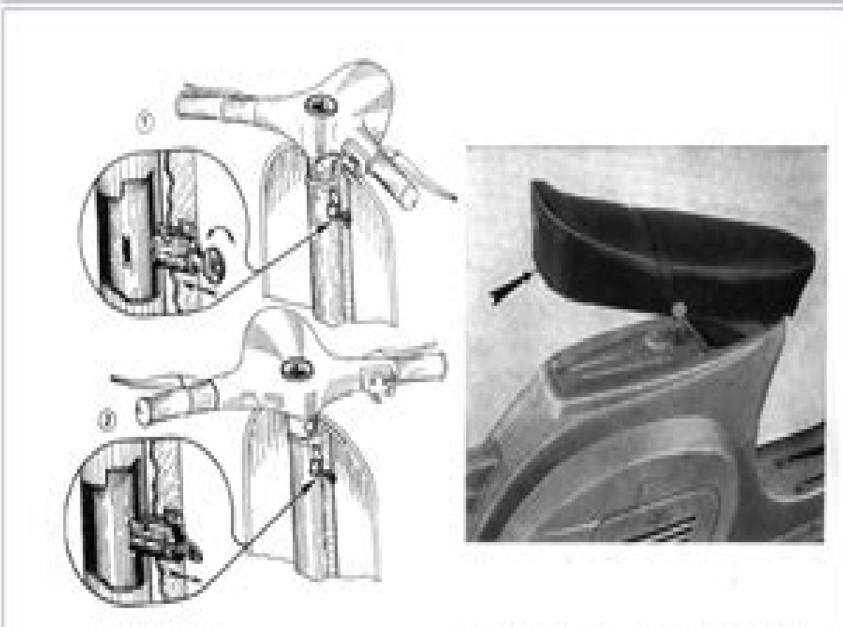
Fig. 4 - Seating lock Fig. 4 - Carrozzina anti - furto 1. Normal position - 2. Locked position 1. Posizione normale - 2. Posizione di blocco
