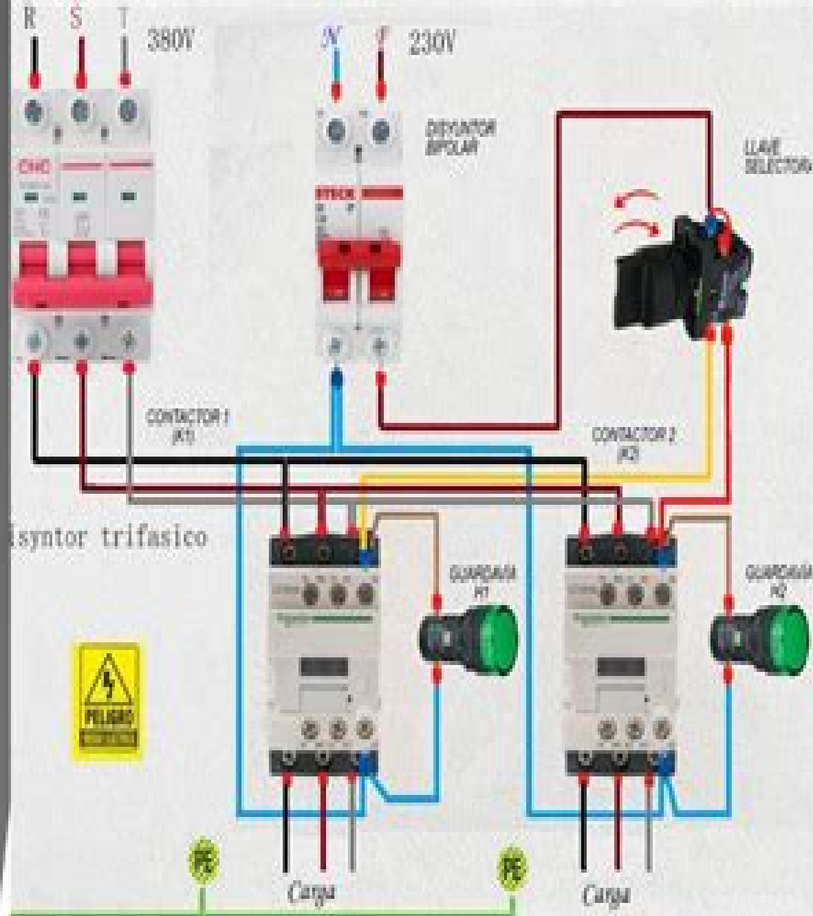
Circuito de mando y selector 3 posiciones para 2 motores
