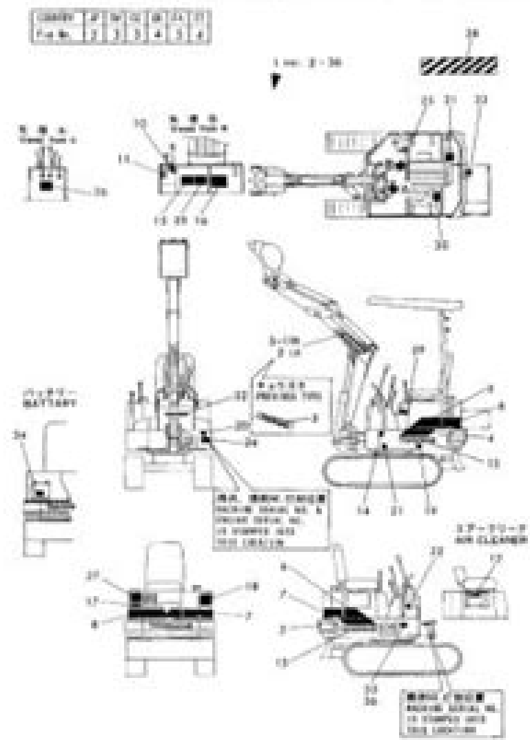
Fig. 5 マイパン (フランス) LABELS (FRANCE SPEC.) SP12, 6106 872121-80128
