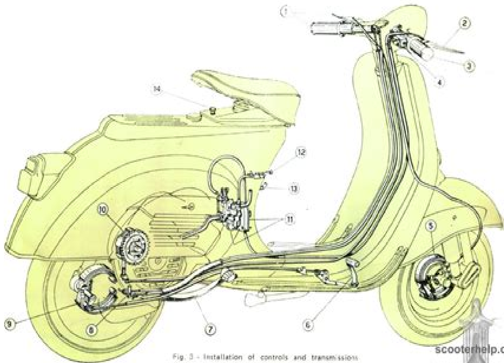
Fig. 3 - Instalación de mandos y transmisiones
