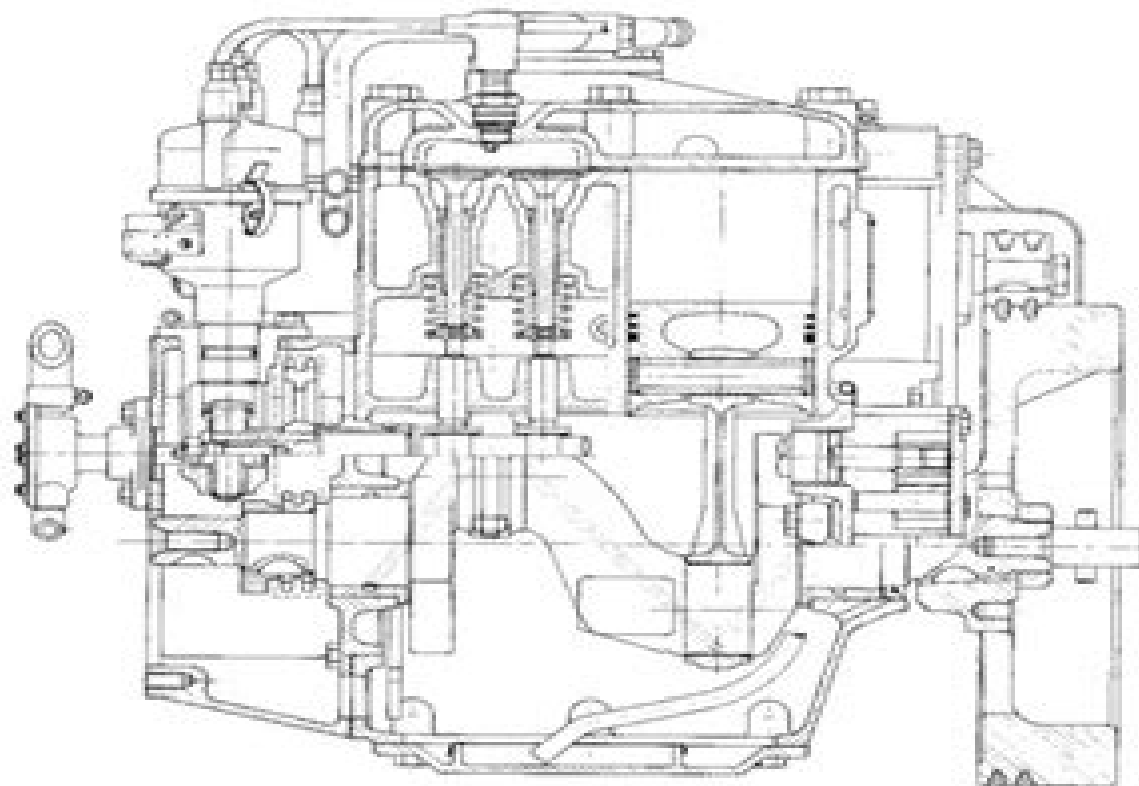
Längdsnitt Longitudinal section
