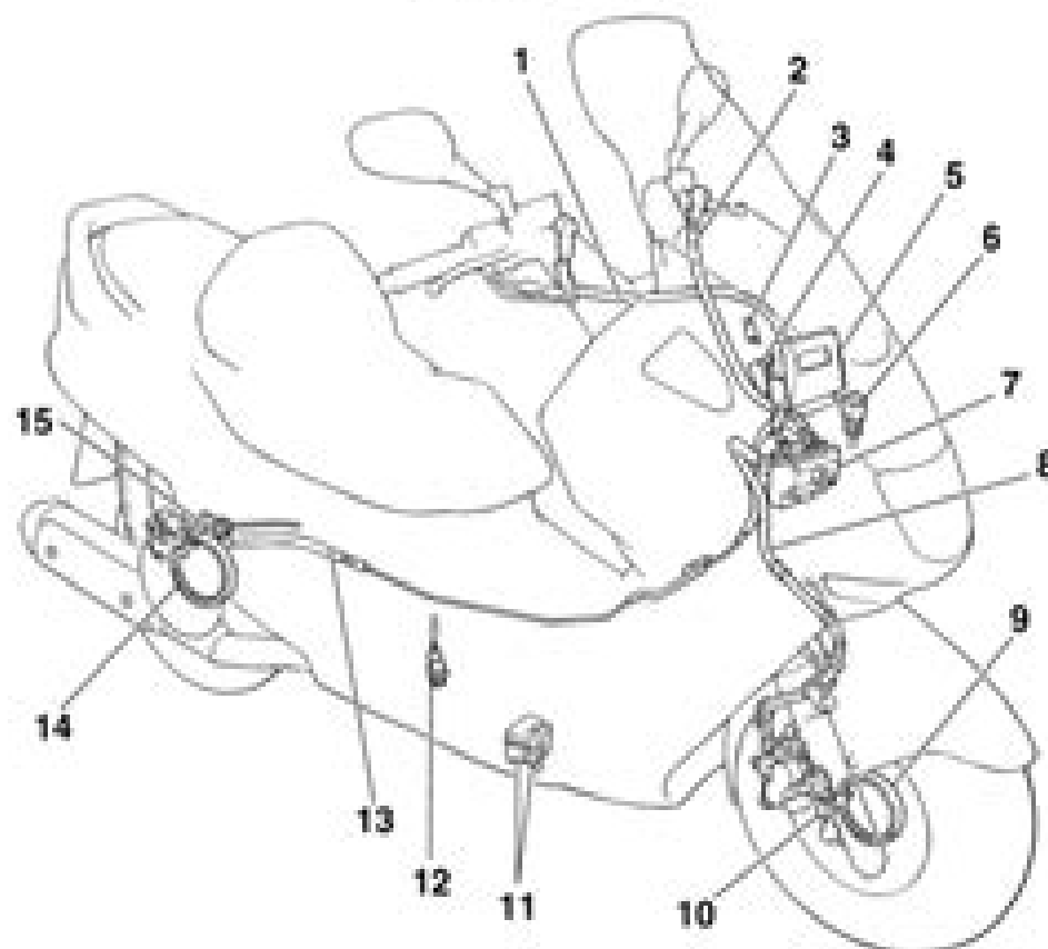
Componenti dell'ABS
