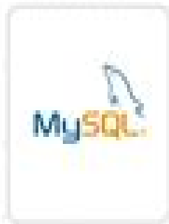
MySQL
