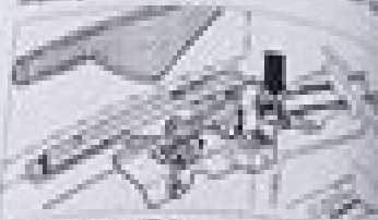
Die Schutzhaube (Pfeil) muss immer gelöst werden, um die Handbremse aus dem Ausparklager zu ziehen.
