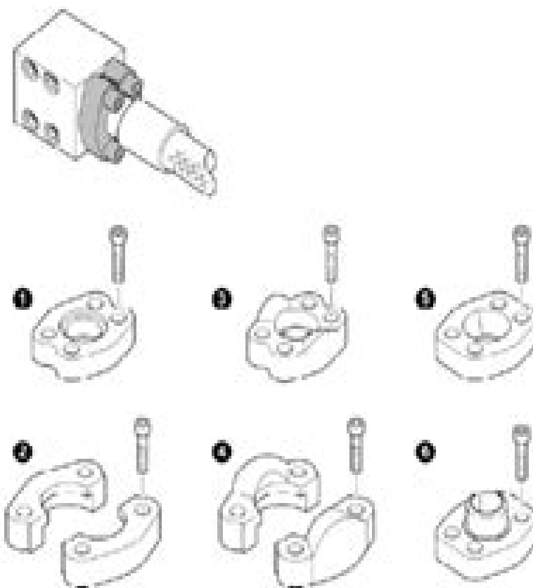
Fig. 1 SAE flanges
